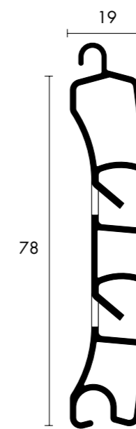
Lüftungsprofil
