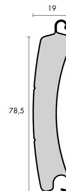
Profil 75
