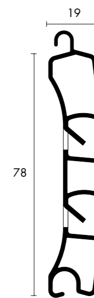
Lüftungsprofil
