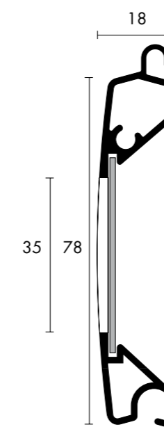
Sichtprofil
