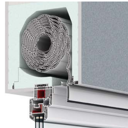
Aufsatz-Element eckig, raumseitig geschlossen für Rollläden – Seite 8
