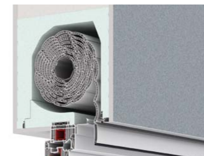
Aufsatz-Element eckig, raumseitig geschlossen für Rollladen – Seite 9
