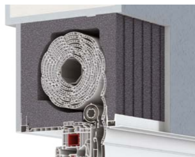
Aufsatz-Element Neo XT für Rollladen – Seite 15
