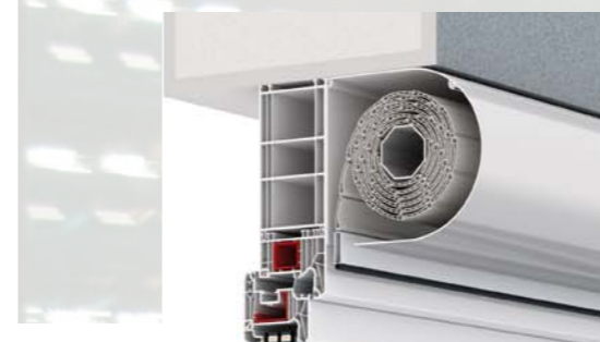
Vorbau-Element rund für Rollladen – Seite 4
