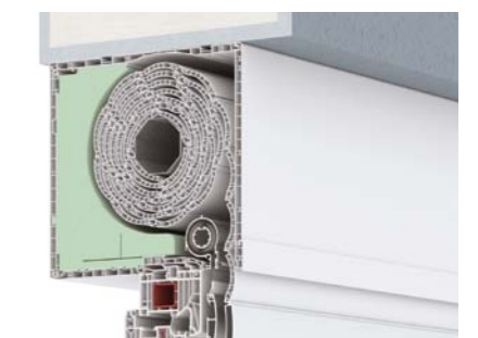
Aufsatz-Element Elite XT für Rollladen – Seite 14
